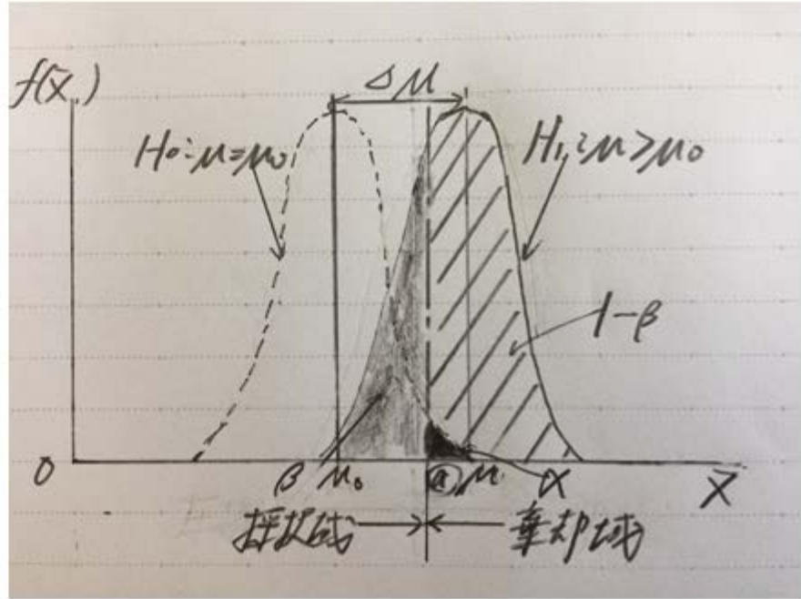
図 2 . \alpha と \beta の関係 ( B )
